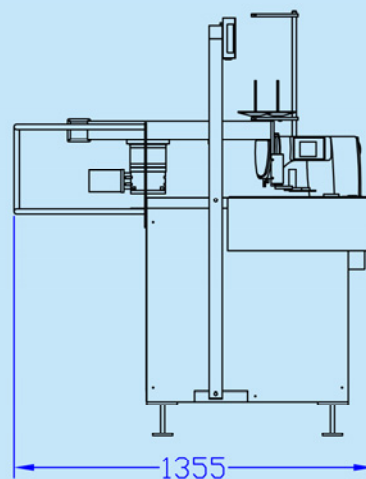
機身外形尺寸圖 Machine external dimensions diagram
